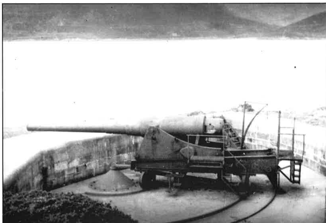
Artillería de Costa - Cañón Krupp de 26cm
